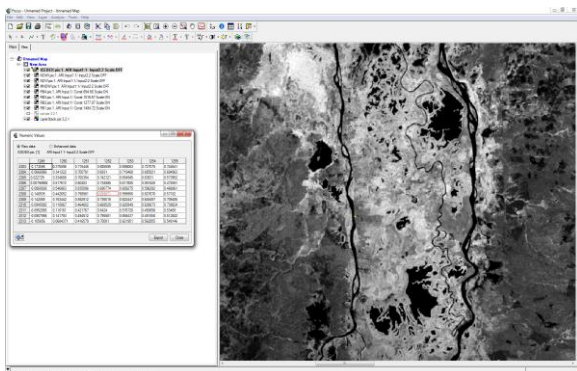
Figura 8. Índice de Agua ICEDEX
