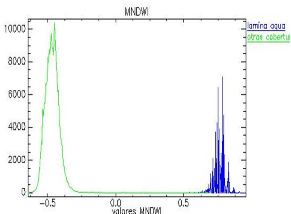
Figura 12. Evaluación de la separabilidad del MNDWI, según el Índice de Fisher
