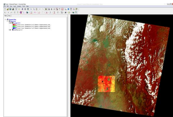
Figura 4. Recorte (Clip) del área de estudio LM5 (Path-Row 854, 1985-03-22)
