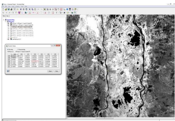
Figura 9. Índice de vegetación normalizado (NDVI)
